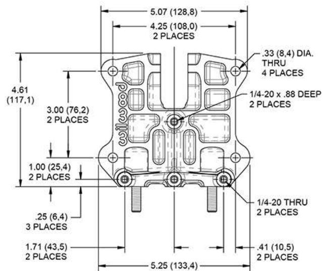
VIEW A-A
